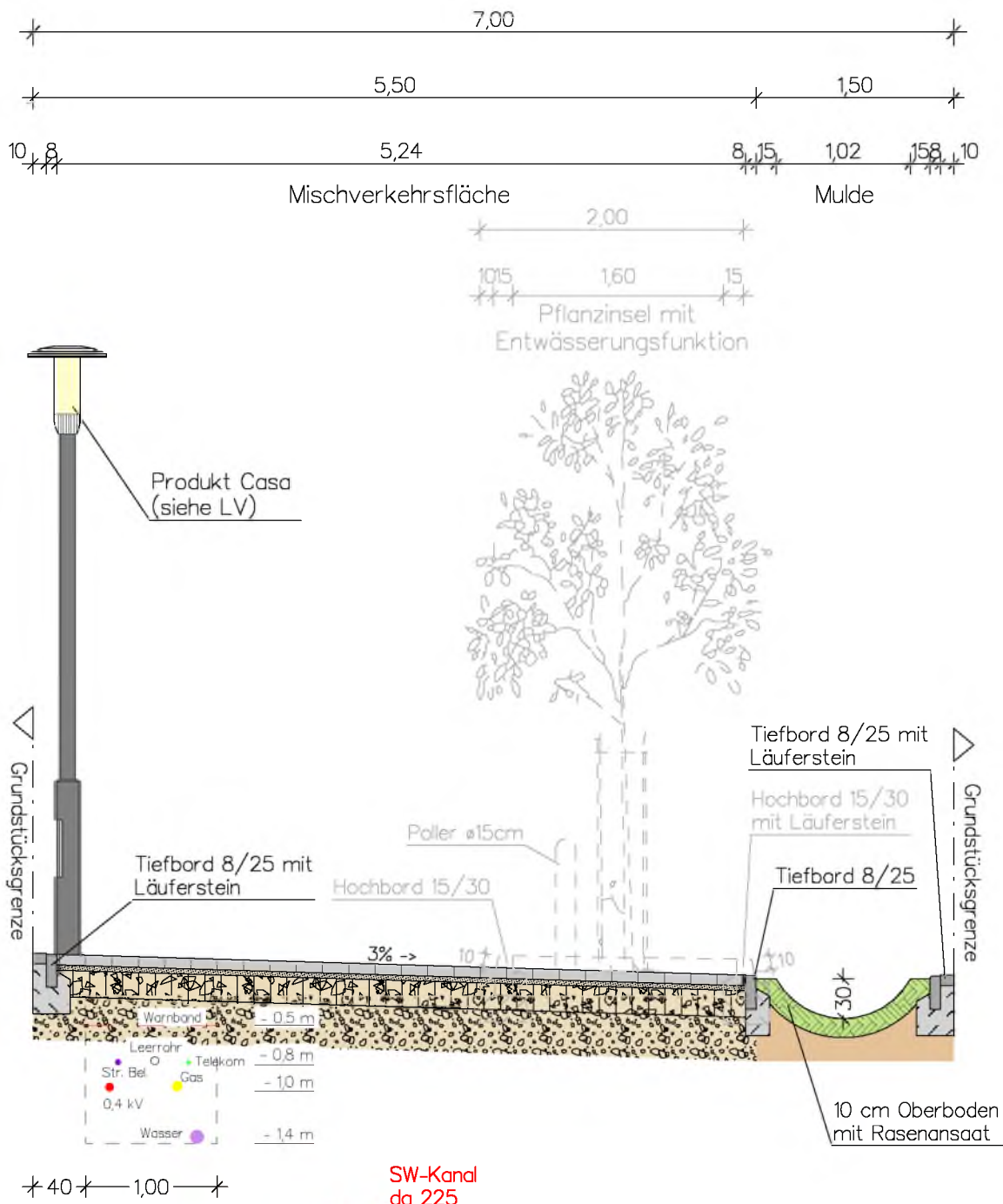
Schnitt B-B
