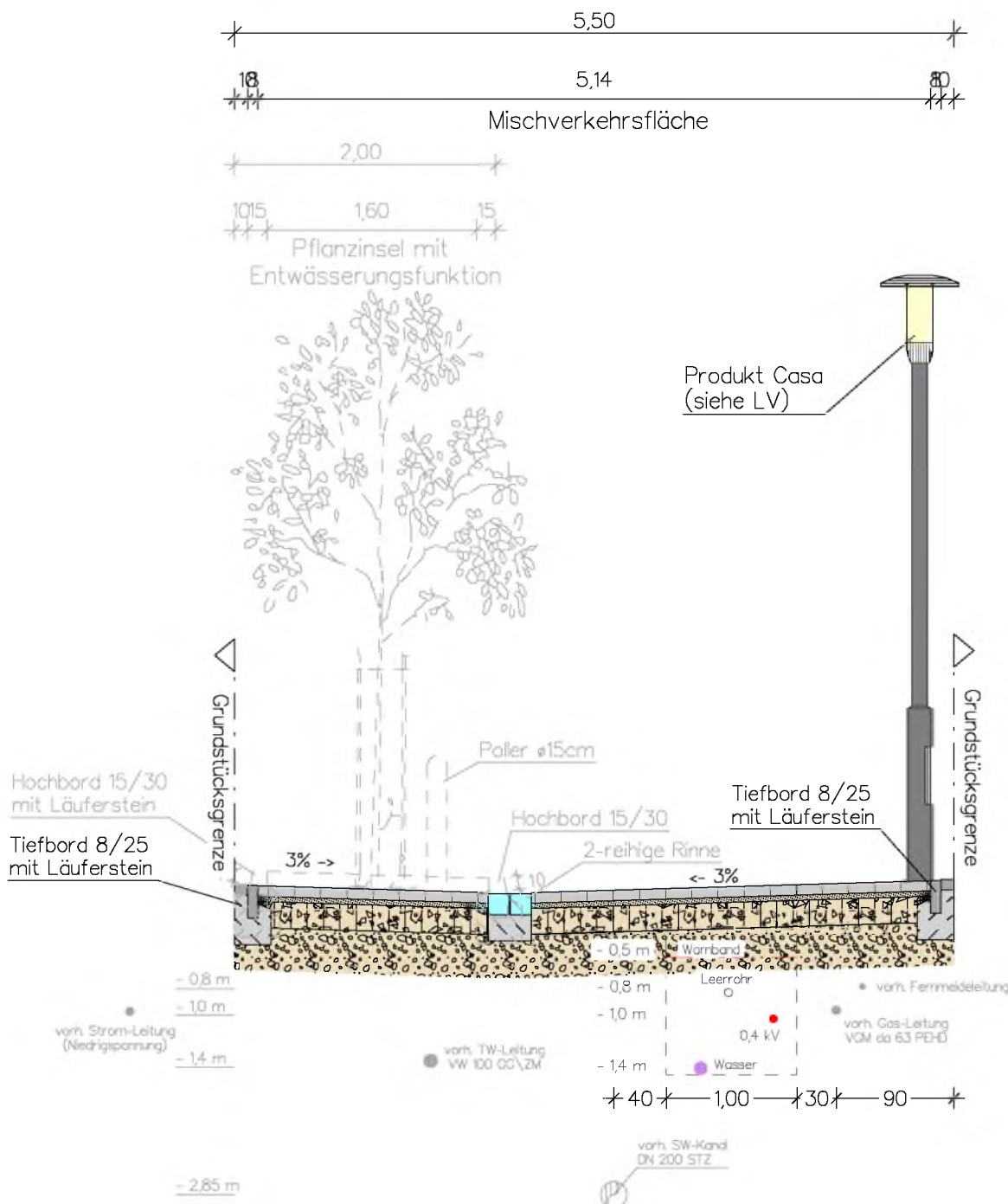
Schnitt C-C
